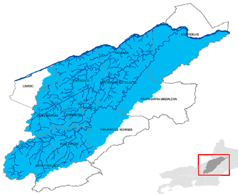
Figura 2 – Região Hidrográfica do Rio Dois Rios. Fonte: INEA
