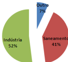
Figura 6 - Participação dos setores usuários por número de empreendimentos no sistema de cobrança, para a RH VII – 2013 (Fonte: INEA)
